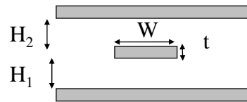
Striplijn
